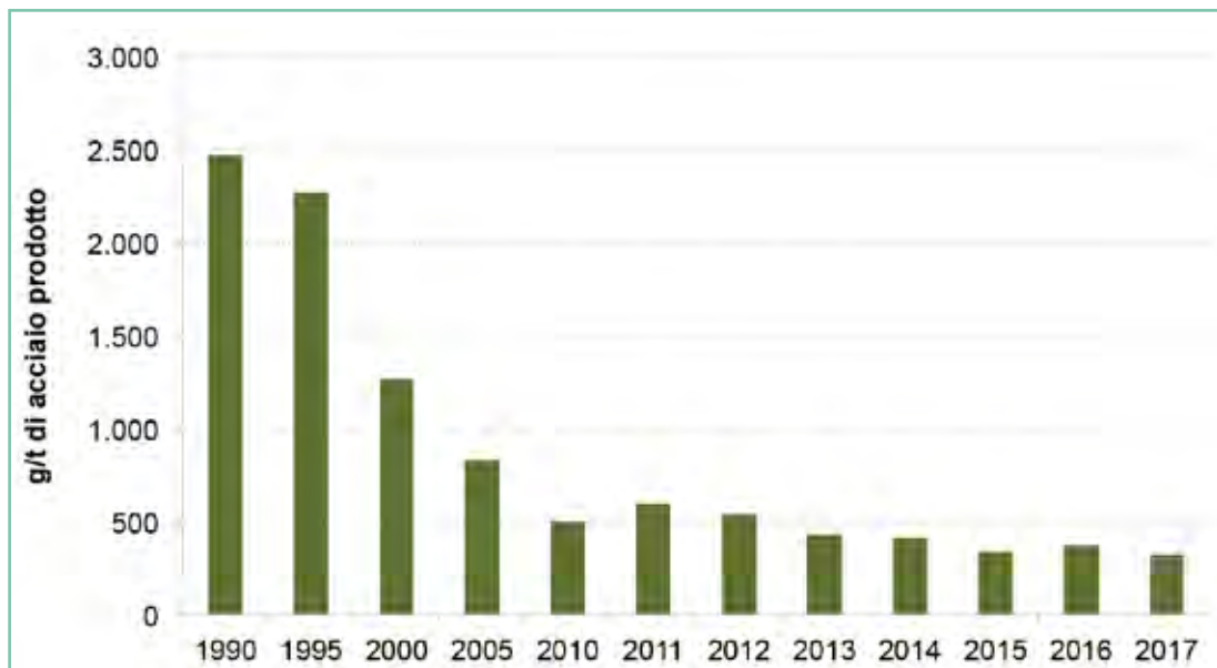
Figura 6.30: Emissioni specifiche di SOx nell'industria siderurgica
