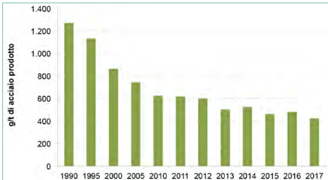
Figura 6.31: Emissioni specifiche di NOx nell'industria siderurgica
