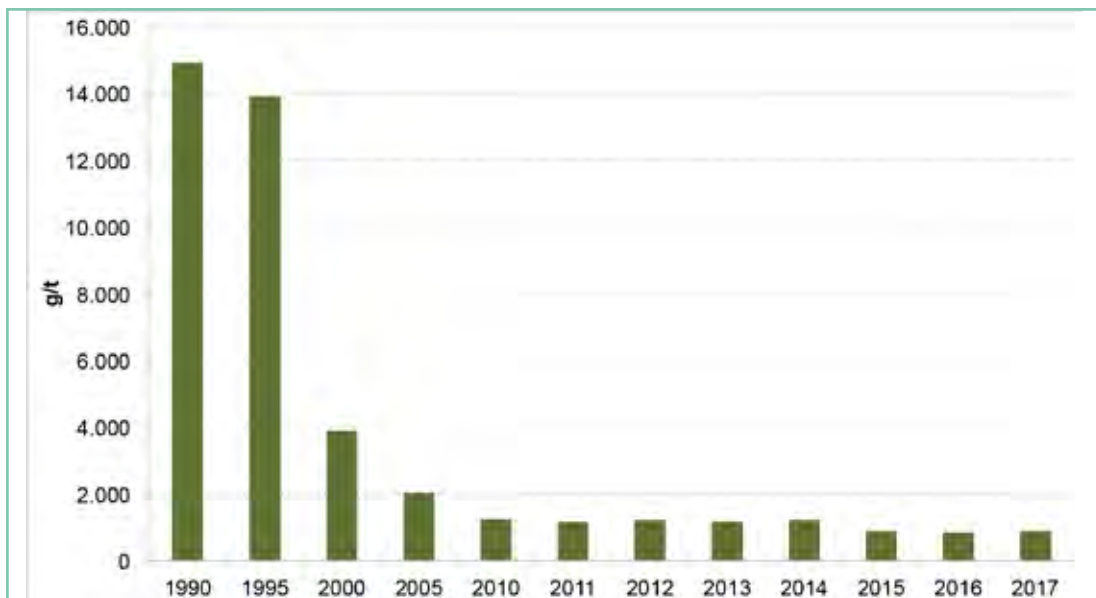
Figura 6.25: Emissioni specifiche di SOx nell'industria chimica
