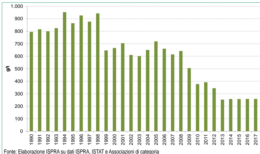
Figura 6.44: Emissioni specifiche di NO x nell'industria dei metalli non ferrosi
