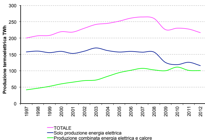
Figura 1.7: Produzione lorda di energia termoelettrica
