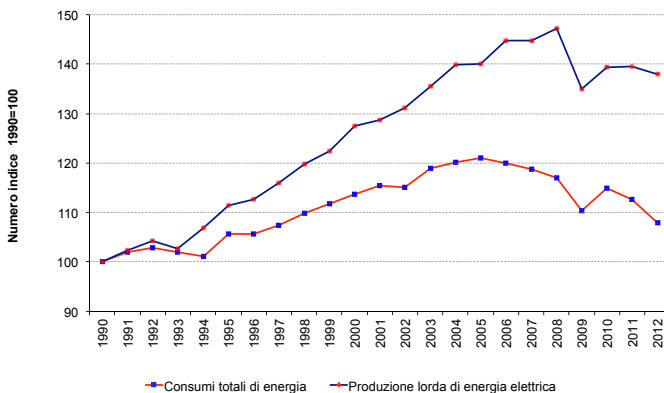
Figura 1.6: Andamento dei consumi totali di energia e della produzione elettrica
