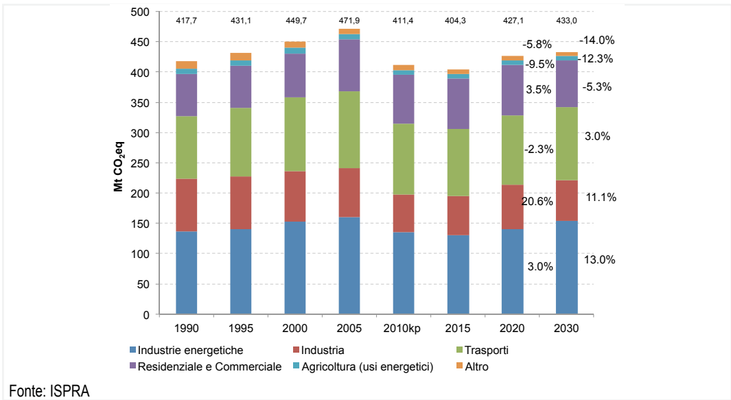
Figura 1.11: Proiezioni delle emissioni di CO 2 eq nei settori energetici (scenario WAM)
