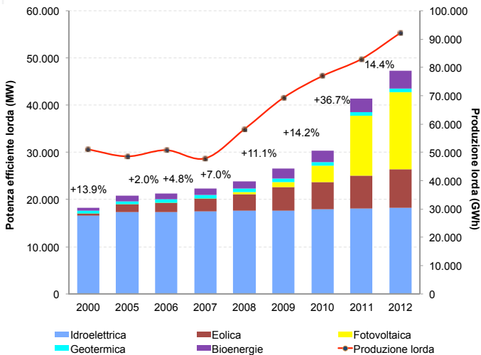
Figura 1.8: Potenza efficiente e produzione lorda degli impianti da fonti rinnovabili
