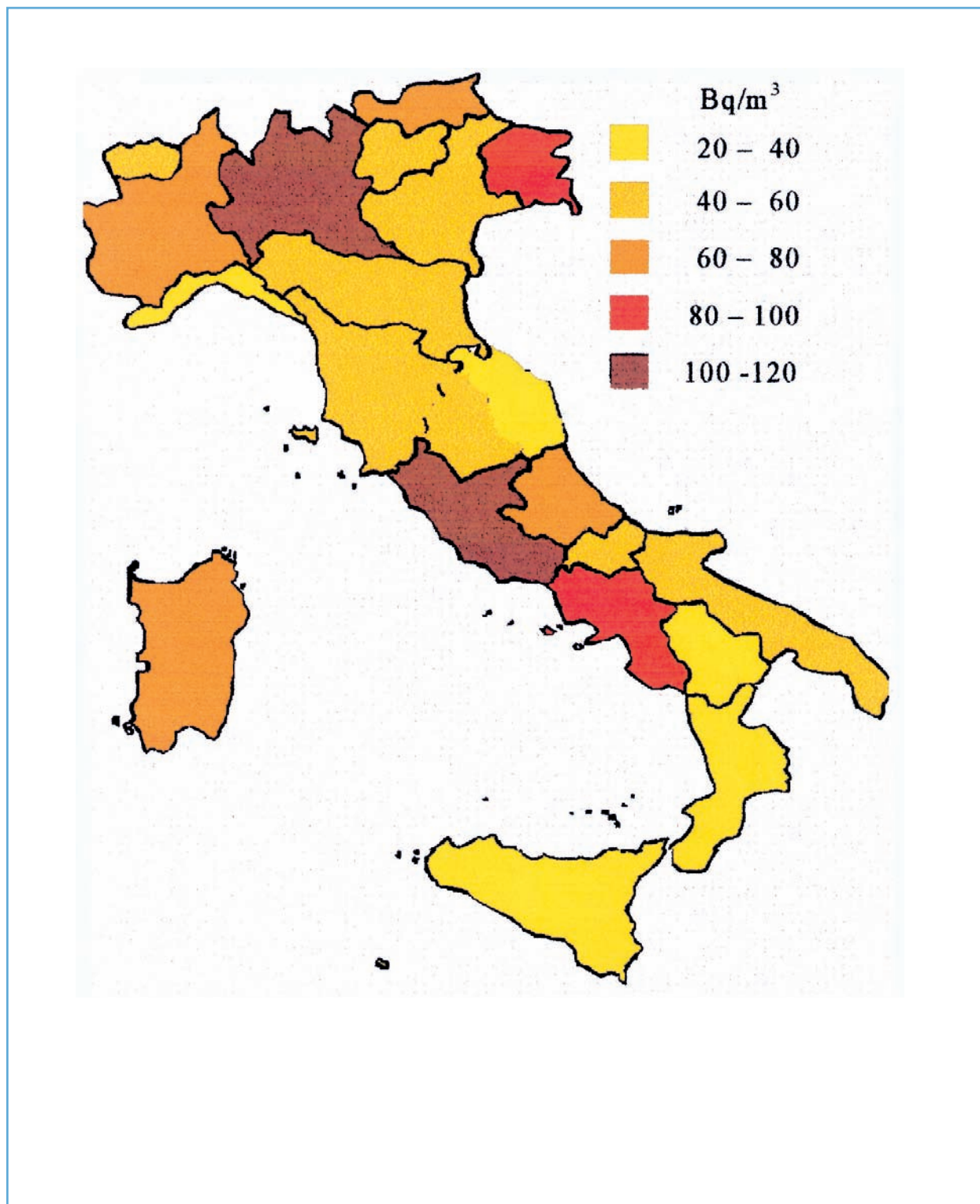
Figura 14.4: Carta tematica per regione e provincia autonoma delle concentrazioni di attività di Rn 222 nelle abitazioni (la scelta degli intervalli ha valore esemplificativo) - Anni 1989-1997
